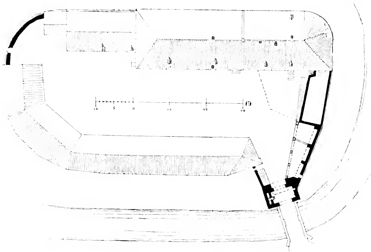
Fig. 28. Angermund. Grundriss der Burg.
